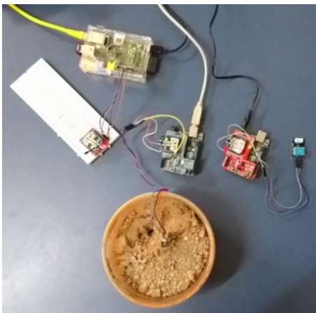
Fig. 4 Rede montada com NPi e dois NAr, sensor DHT11 e Higrômetro.
