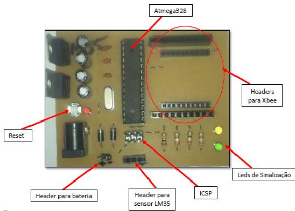
Fig. 3 NAr prototipada para sensor LM35
