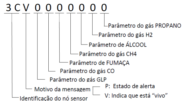
Fig. 2 Mensagem enviada pelo NAr com MQ-2.
