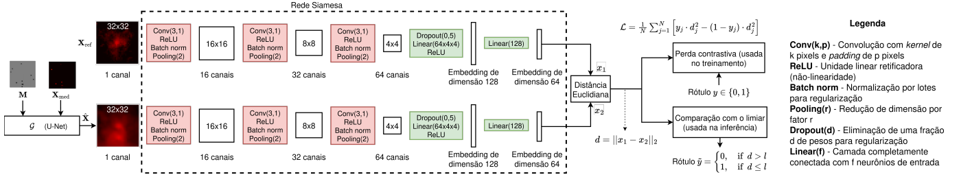
Fig. 2: Rede siamesa para comparação entre dois REMs. As camadas são representadas pelos retângulos coloridos, cujos detalhes são apresentados na legenda, à direita. A mesma rede é reutilizada para ambas as matrizes de entrada.
