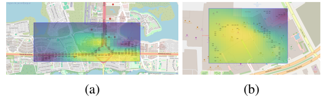
Fig. 3: Potência interpolada nas ROIs 1 e 2 por Kriging. Os números indicam a potência média nos pontos medidos.
