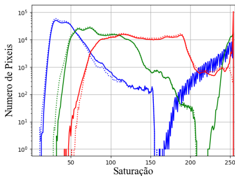
Fig. 2. Histograma contendo imagem original (linhas pontilhadas) e imagem processada (linhas contínuas).
