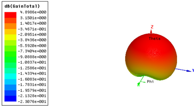
Fig. 8. Diagrama de Radiação para uma DRA de FNT0 adicionada de 16% de ZnO.
