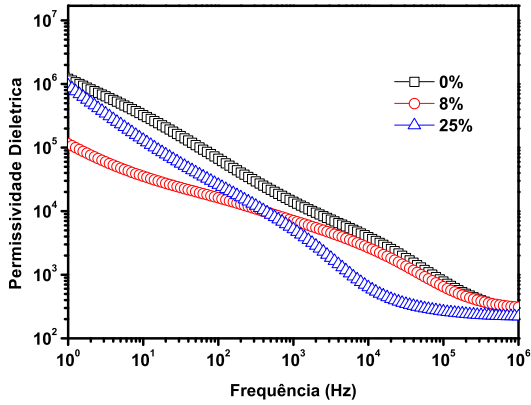
Fig. 2. Efeito do ZnO na permissividade dielétrica do FNTO.
