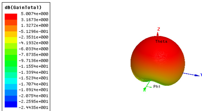
Fig. 9. Diagrama de Radiação para uma DRA de FNT0 adicionada de 25% de ZnO.
